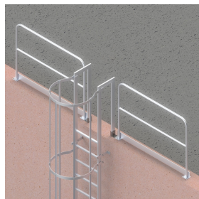
Garde-corps de sortie
