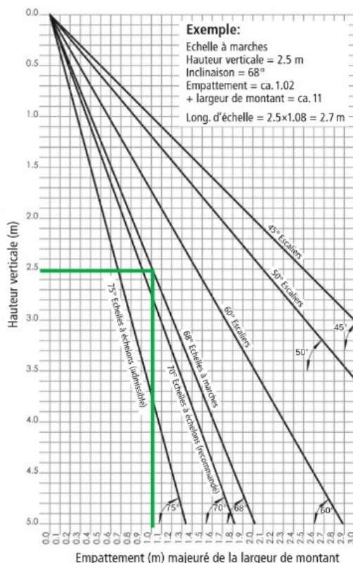
Diagramme pour le calcul de l'empattement
